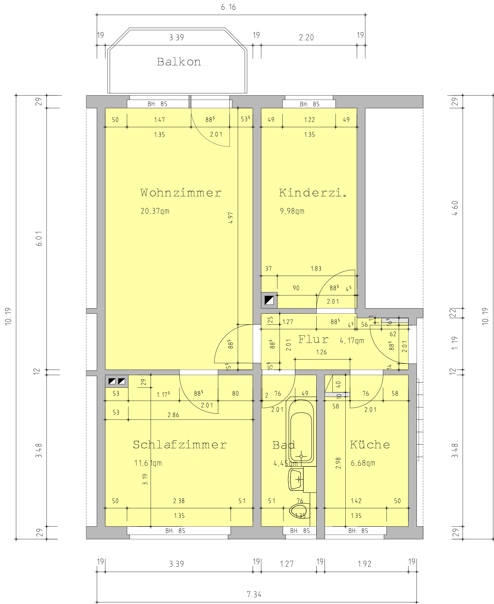
Grundriß Wohnung C – EG bis 3.OG, M 1:50
